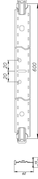
Поперечная направляющая 15/29 L=600
